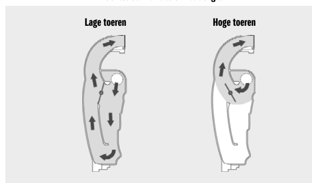
Luchtstroomvariabele inlaatlengte
